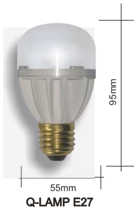
Q-LAMP E27
